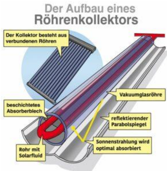
Abbildung 28: Aufbau eines Röhrenkollektors
